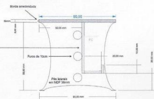
Mesa - Vista Lateral
